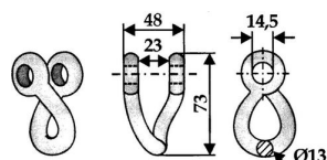
Gedrehter Schäkel 73x48mm
